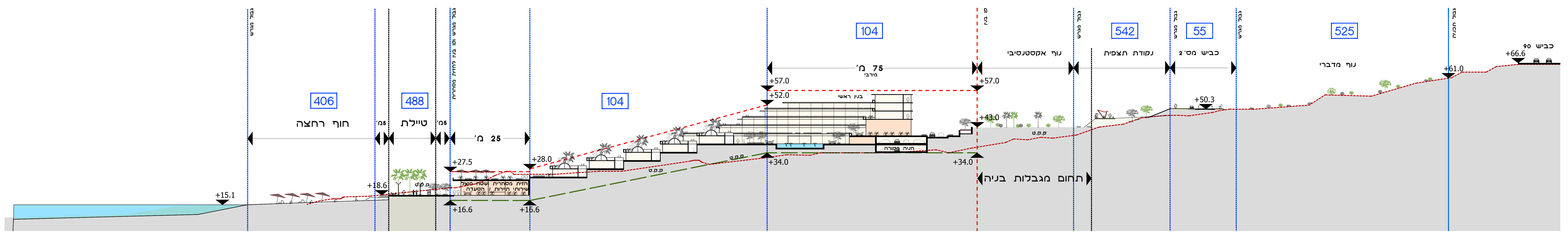
חתך ב-2
